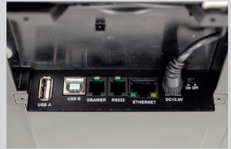
Conexiones: USB-A, USB-B, cajón monedero (DRAWER), RS232, Ethernet, Alimentación, ON/OFF
